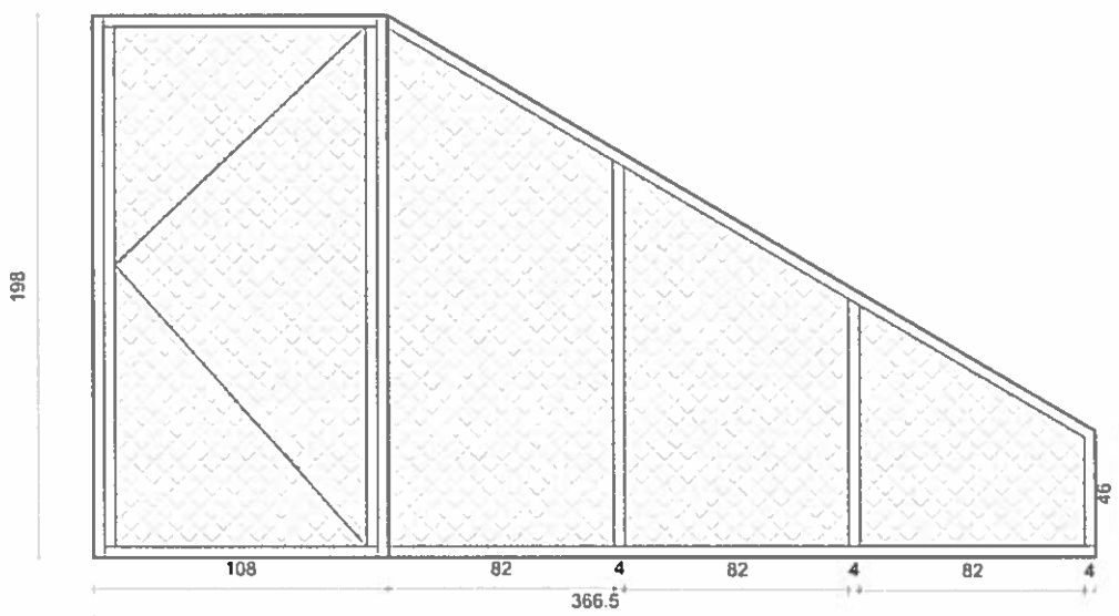
WIDOK ZABUDOWY Z SIATKI
